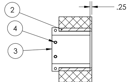
SECTION D-D SCALE 1 : 6
